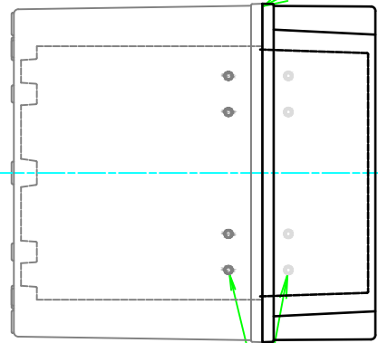
ヒンジガイドマーク Guide markings for Hinge
