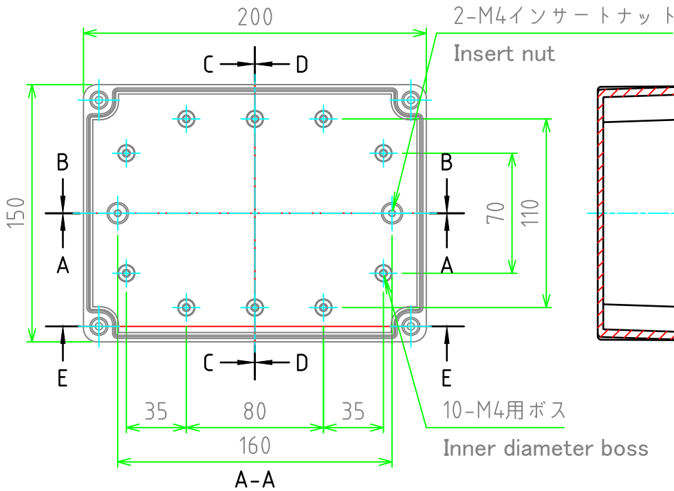
ボディー (内視) Body (Internal View)
