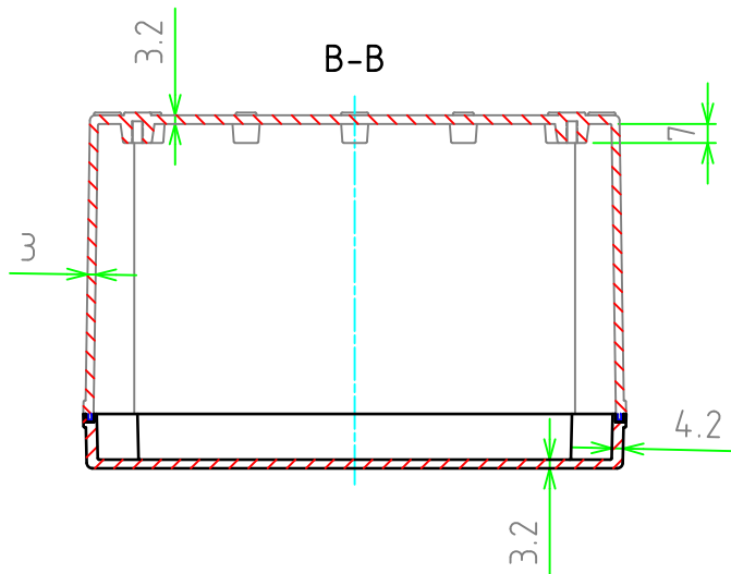
ボディー(内視) Body (Internal View)
