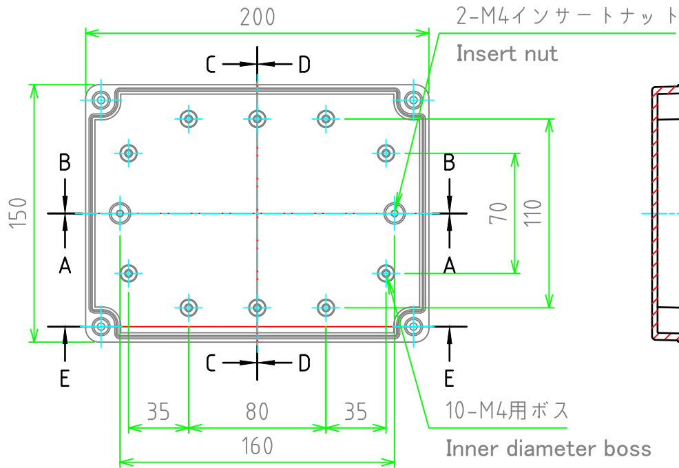
ボディー(内視) Body (Internal View)
