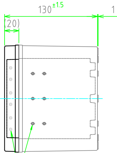
ラッチガイドマーク Guide markings for Latch
