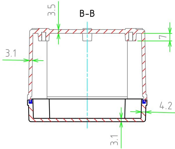
ボディー(内視) Body (Internal View)
