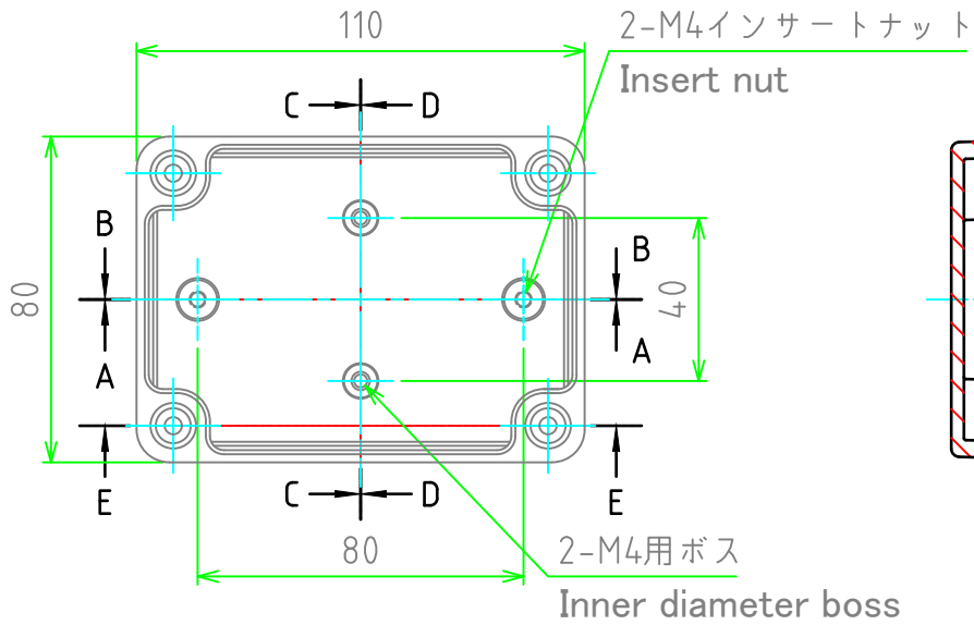
ボディー(内視) Body (Internal View)
