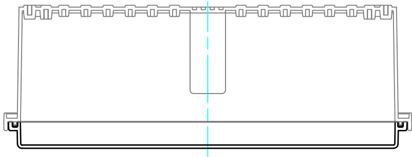
ボディー(内視) Base (Internal View)
