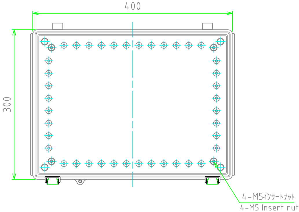
ボディー(内視) Base (Internal View)
