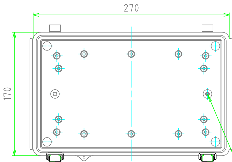
ボディー(内視) Base (Internal View)
