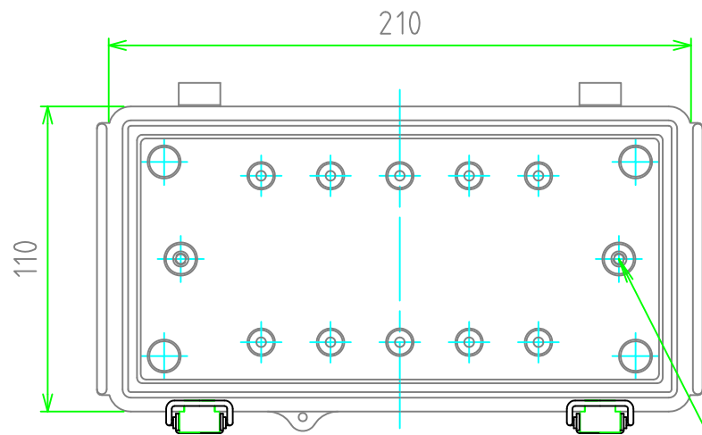
ボディー(内視) Base (Internal View)
