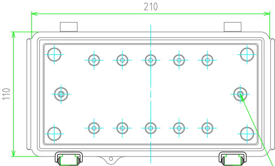
ボディー(内視) Base (Internal View)
