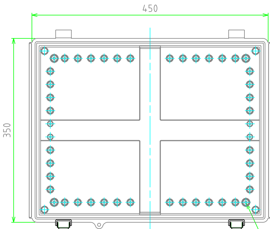
ボディ(内視) Base (Internal View)
