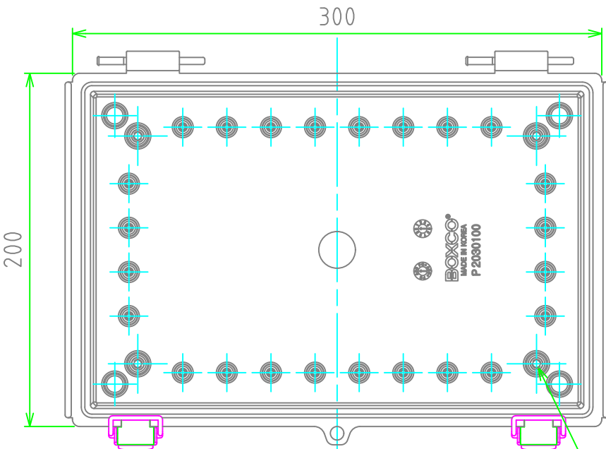
ボディー(内視) Base (Internal View)
