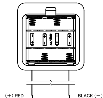
電池ボックス内部 Battery box
