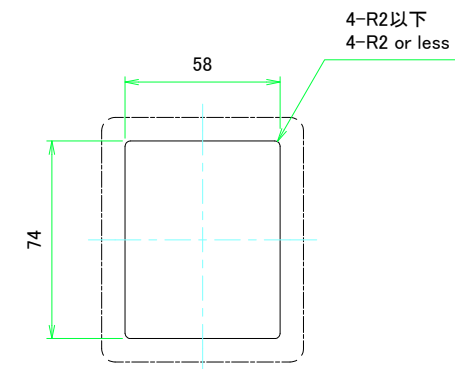
取付穴加工図 Mounting hole
