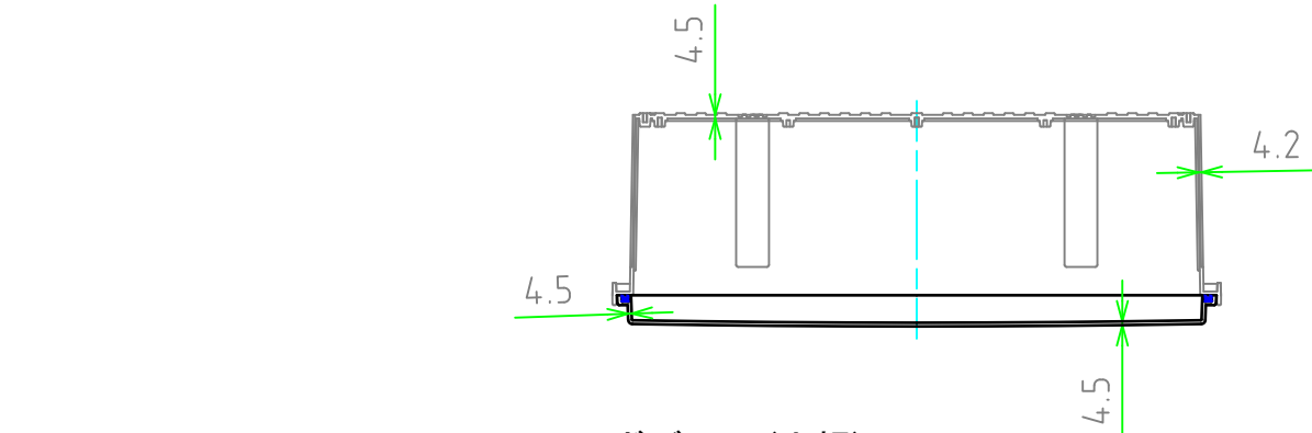
ボディー(内視) Base (Internal View)
