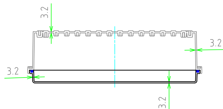
ボディ (内視) Base (Internal View)
