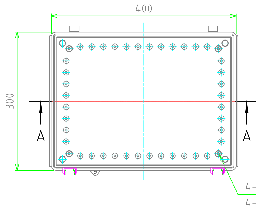
ボディ (内視) Base (Internal View)
