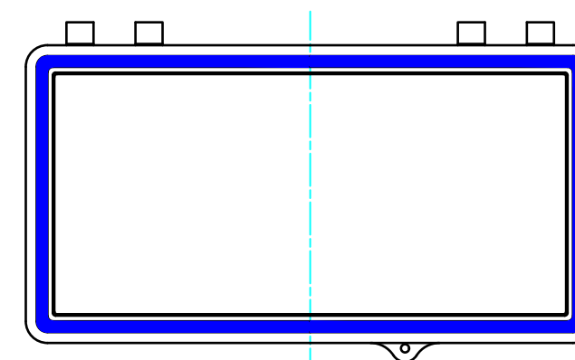
4-M4タッピングビス用ボス 4-Boss for M4 tapping screw
