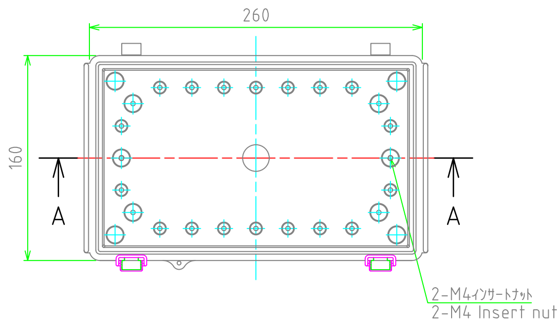
ボディー(内視) Base (Internal View)
