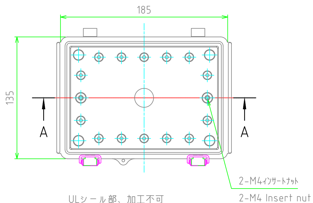
ボディー(内視) Base (Internal View)
