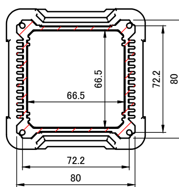
A-A (1:2.5)
