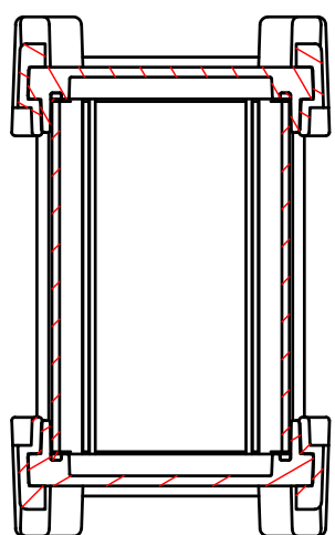
B-B (1:2.5)
