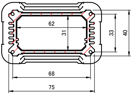
A-A (1:2)
