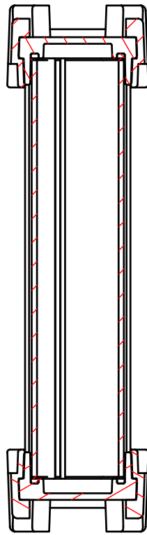
B-B (1:2)
