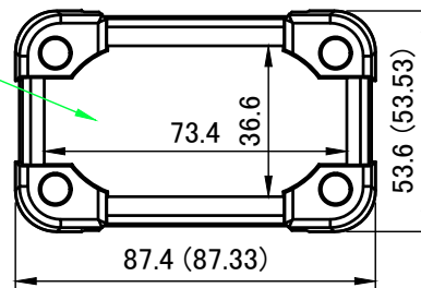
A-A (1:2)
