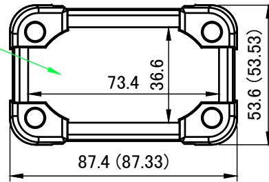
A-A (1:2)
