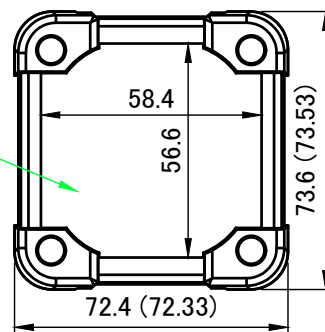
A-A (1:2)
