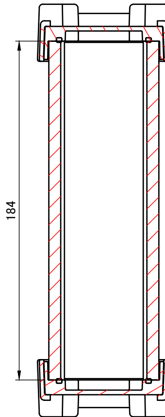
C-C (1:2)
