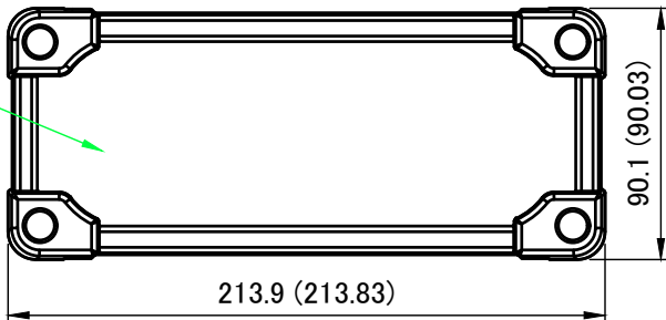
A-A (1:3)
