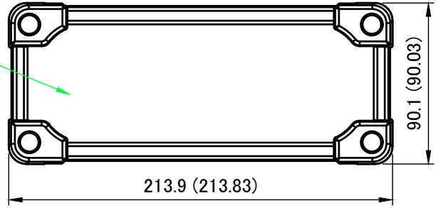
A-A (1:3)
