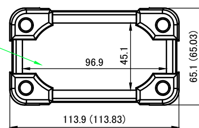
A-A (1:2.5)
