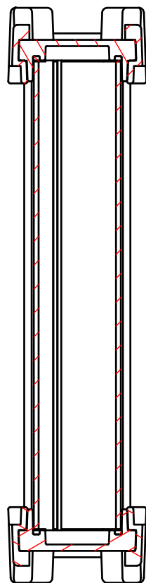
B-B (1:2.5)
