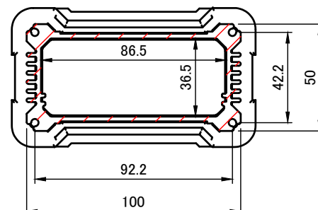
A-A ( 1 : 2.5 )
