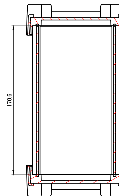
C-C ( 1 : 2.5 )
