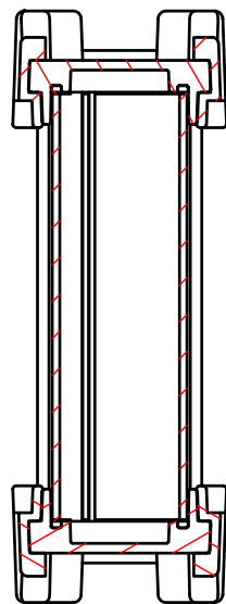
B-B (1:2.5)
