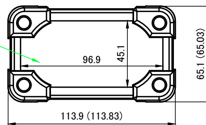
A-A (1:2.5)
