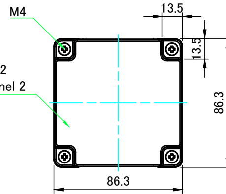
A-A ( 1 : 2.5 )
