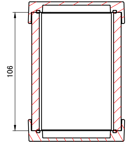
C-C (1:2)
