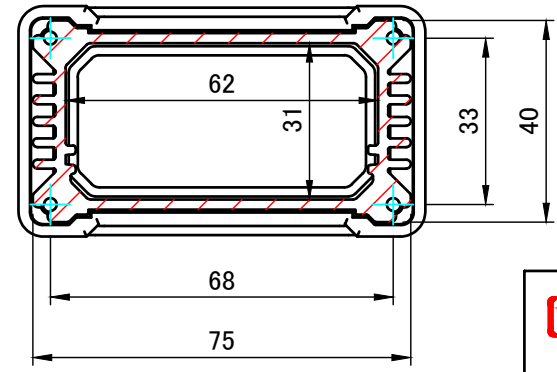
A-A ( 1 : 1.5 )
