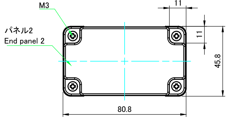
A-A ( 1 : 1.5 )
