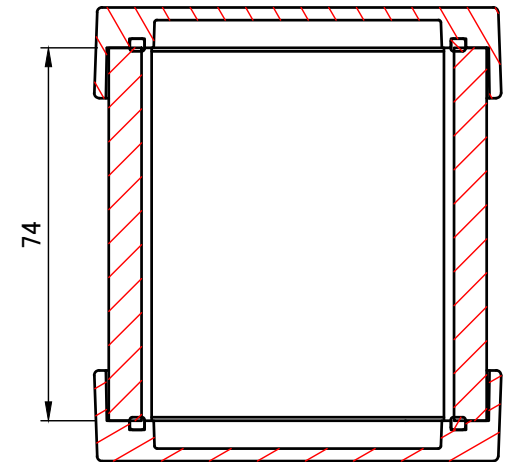
C-C ( 1 : 1.5 )
