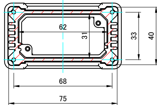
A-A (1:1.5)
