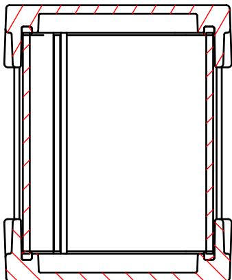
B-B ( 1 : 1.5 )
