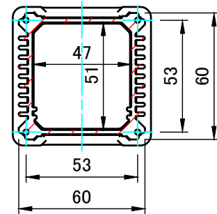
A-A ( 1 : 2.5 )
