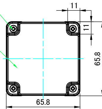
A-A (1:2)
