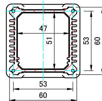
A-A (1:2)
