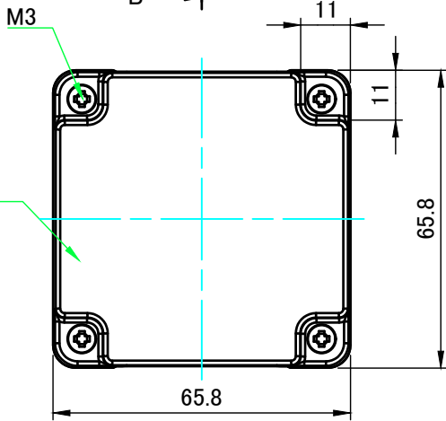
A-A ( 1 : 1.5 )
