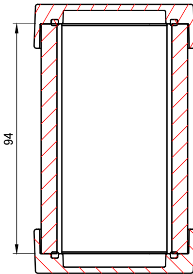
C-C ( 1 : 1.5 )
