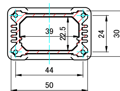
A-A ( 1 : 1.5 )
