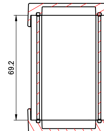
C-C ( 1 : 1.5 )
