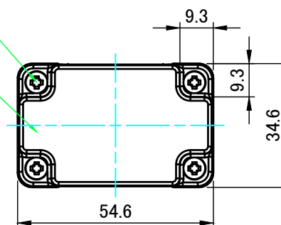
A-A ( 1 : 1.5 )
