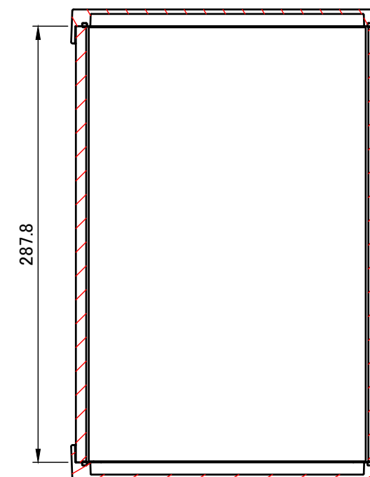
C-C ( 1 : 3.5 )
