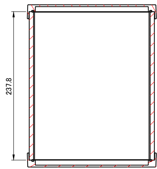
C-C ( 1 : 3.5 )
