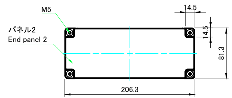
A-A ( 1 : 3.5 )
