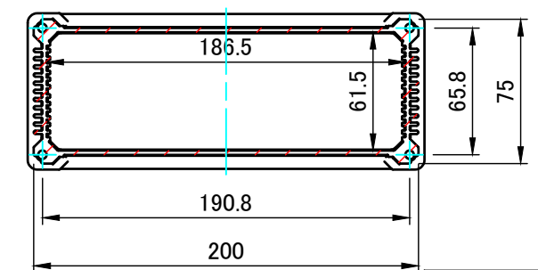
A-A ( 1 : 3.5 )
