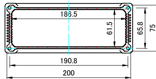
A-A ( 1 : 3.5 )
