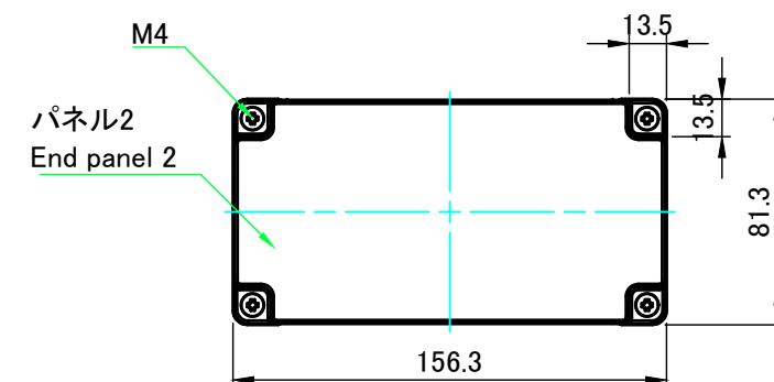
A-A (1:3)
