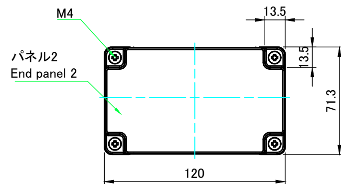
A-A ( 1 : 2.5 )
