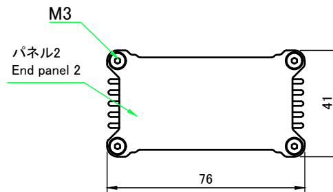
A-A ( 1 : 2 )
