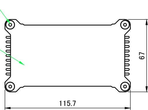
A-A (1:2)
