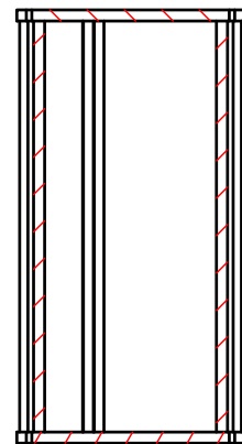
B-B ( 1 : 1.5 )
