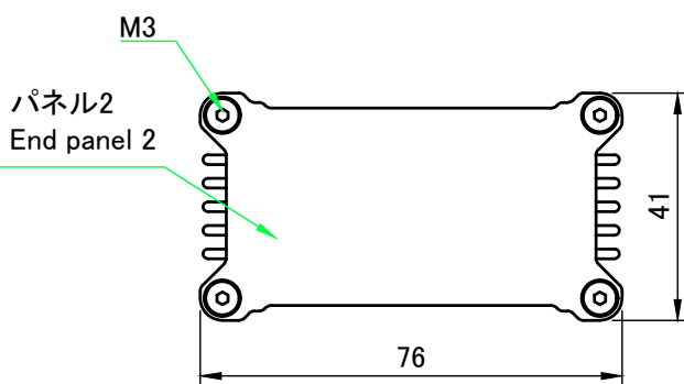
A-A ( 1 : 1.5 )
