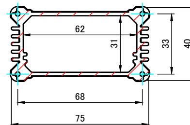
A-A ( 1 : 2 )
