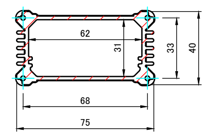
A-A ( 1 : 2 )
