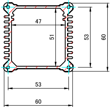
A-A ( 1 : 2 )
