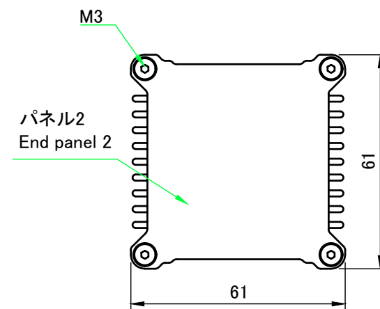
A-A ( 1 : 1.5 )
