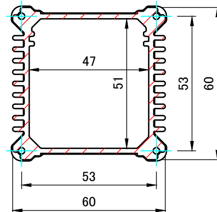
A-A ( 1 : 1.5 )
