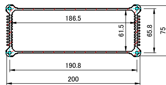
A-A ( 1 : 3.5 )
