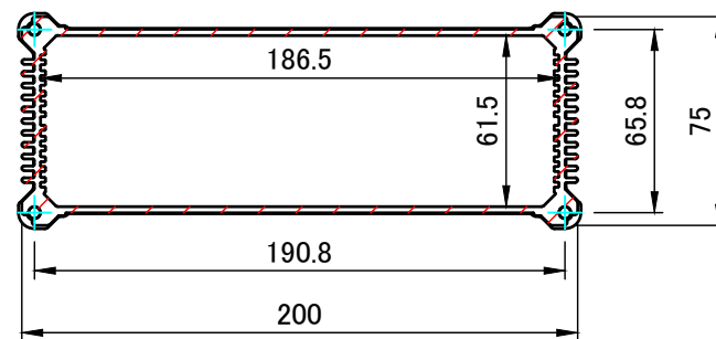
A-A (1:3)
